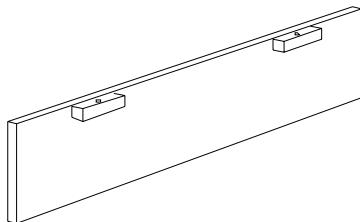
P5 - End Apron (1)
